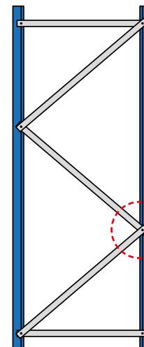
Kreuzungspunkt Rahmenfachwerk
